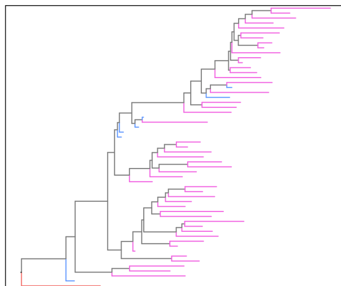
NA Subtree 2
