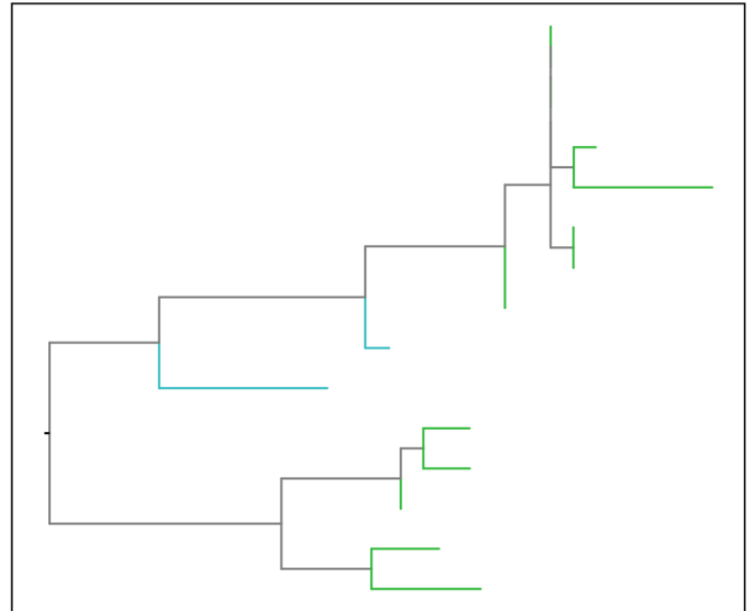
NS1 Subtree 2
