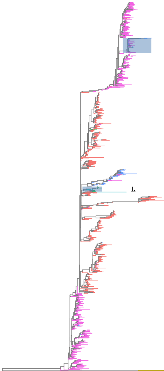
NS1 Tree
